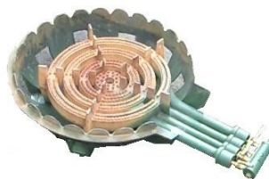
4連コンロ(LPG) サイズ: W540 × D740 × 170 重量: 約21kg ガス消費量: 約1.37kg/h ※使用時はベニヤ板などを敷いてご使用ください
